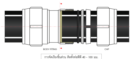
การจัดเรียงชิ้นส่วน ติดตั้งท่อพีพี 40 - 100 มม.
